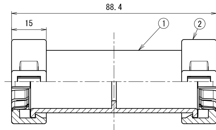
A-A断面図
